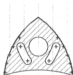
COFAS DE MACHOS DE MAYOR Y DE TRINQUETE
